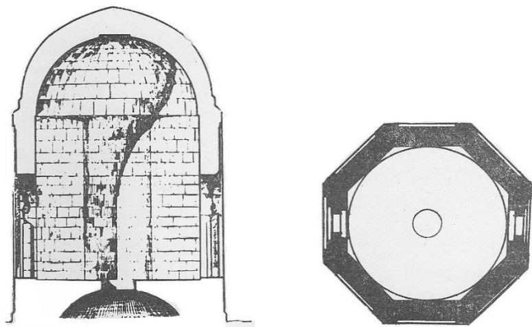
Şəkil 3. Şeyx Babı xanəgahında səkkiztilli türbənin planı və kəsiyi
